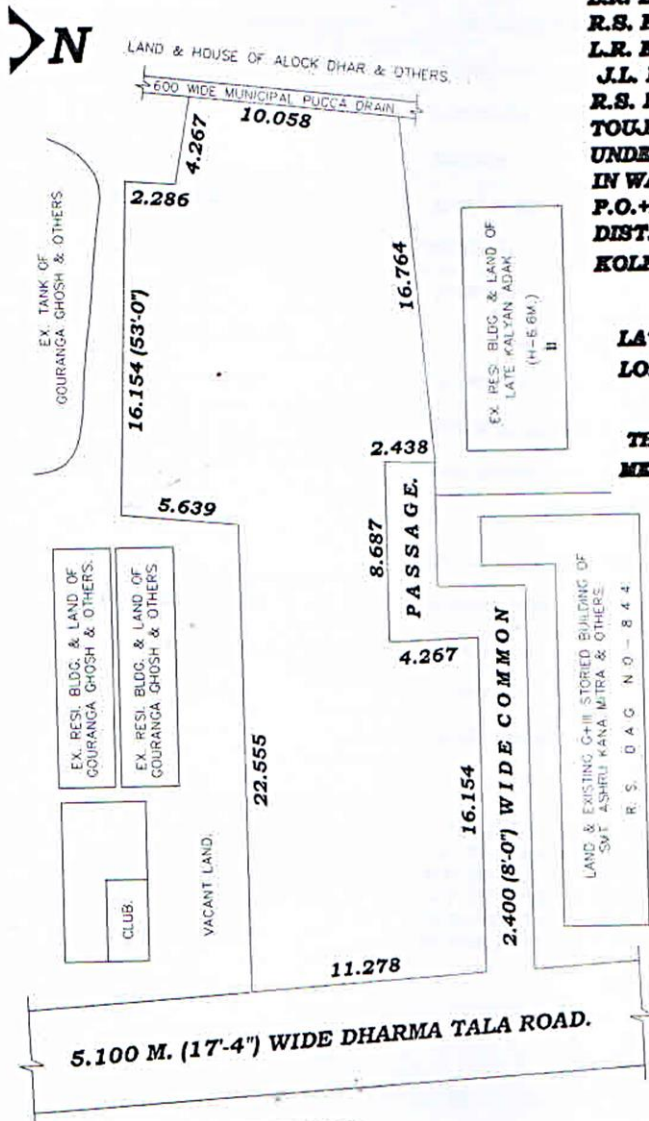
SITE PLAN.
